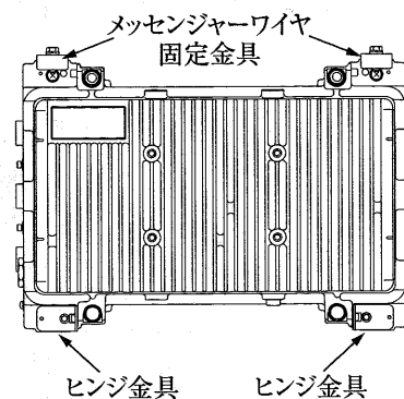
通常時の接続
