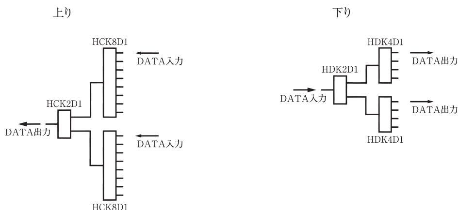
図-5 システム図
