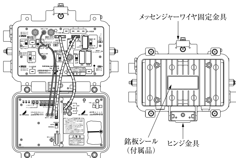
入出力反転時の接続
