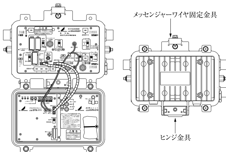
通常時の接続
