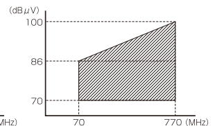
図2. TILT入力
