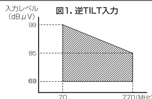
図1. 逆TILT入力
