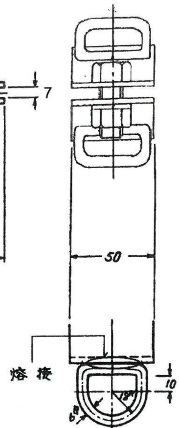
4方環取付詳細図 S=1/2
