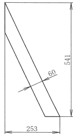
リブ詳細 t6
