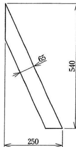
リブ詳細 t6
