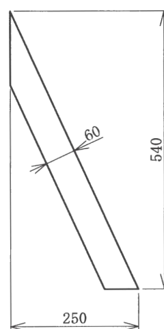
リブ詳細 t6
