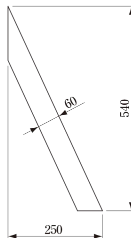
リブ詳細 t6
