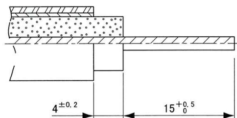
ケーブル切出し寸法
