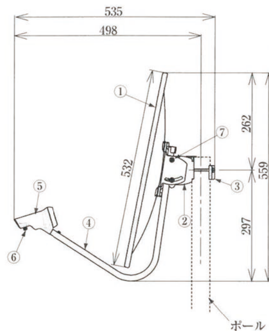
側面
