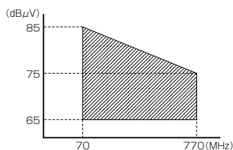
図1. 逆TILT入力 (W30L1C, W30L2C, F30L1C)
