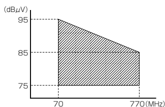
図2. 逆TILT入力 (F20L1C)
