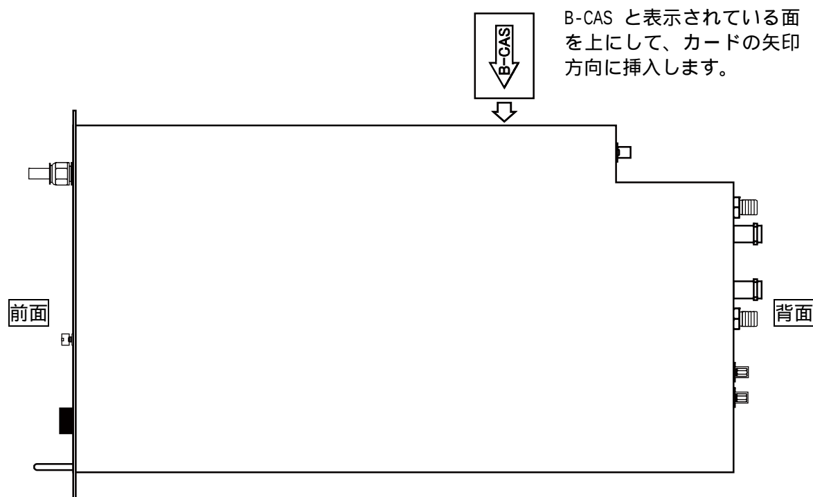
図 6-2 B-CAS カード装着方法
