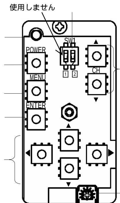
図 5-3 チューナー部
